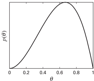
Beta(3,2)
