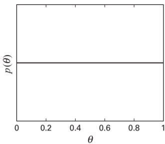
Beta(1,1)
