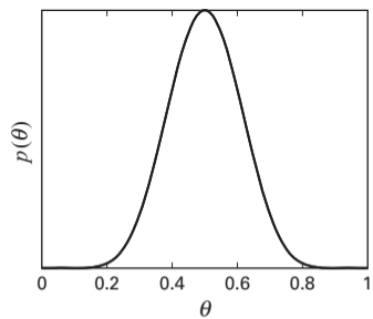
Beta(10,10)
