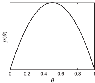
Beta(2,2)
